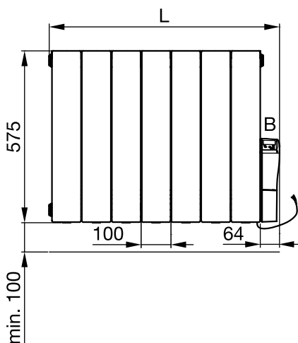
Vorderansicht, ALE
