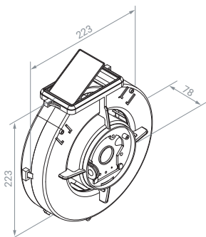
Lüftereinsatz
