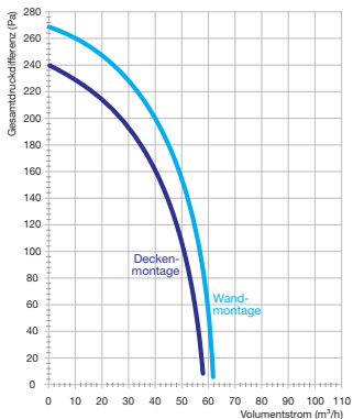
Unterputzlüfter
