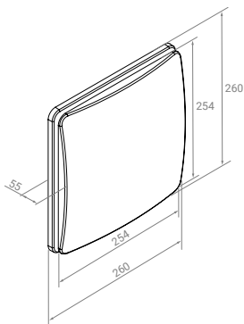
Lüfterfassade
