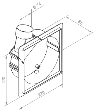
Lüfterfassade
